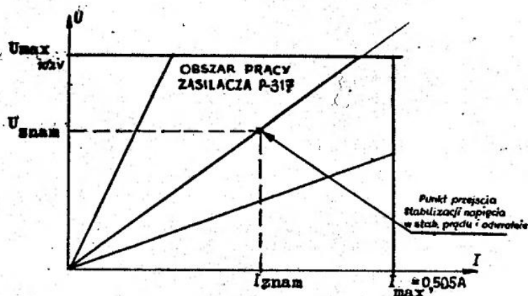
Rys. 1. Obszar pracy zasilaczy P - 316, P - 317 / dla P - 316 U_{maksymalne} = 51 \text{ V} , I_{maksymalne} = 1 \text{ A} /
