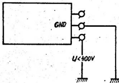
Rys. 5. Przyłożenie napięcia względem masy zasilacza.
