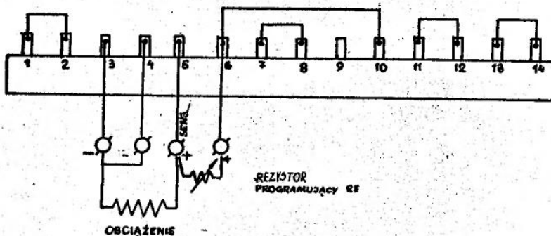
Rys. 11. Układ programowania prądu wyjściowego rezystorem zewnętrznym.
